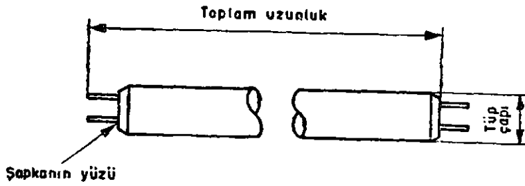
ŞEKİL : 1a — Tüp biçimli lamba boyutlarının ölçüleceği yerler
