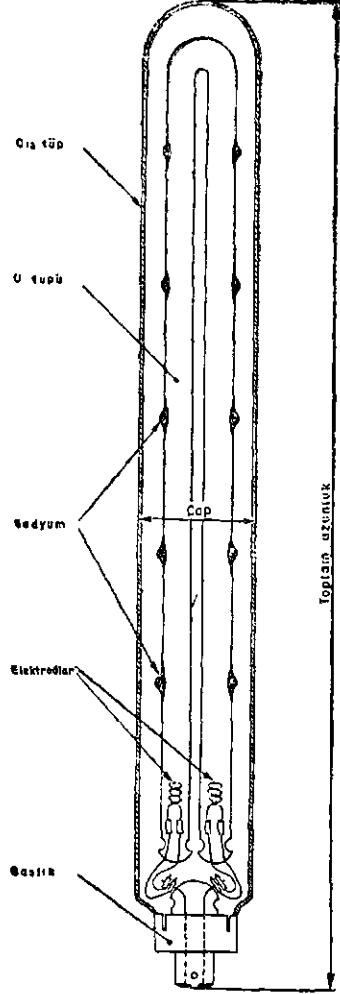
ŞEKİL : 1 — U - biçimli sodyum buharlı boşalmalı lamba
