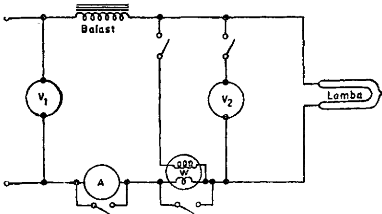
ŞEKİL : 2 — U biçimli lamba deneyleri için devre şeması
