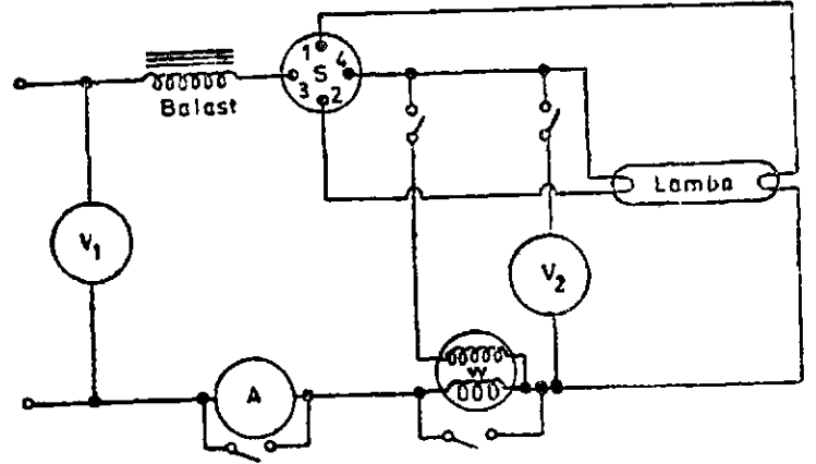
ŞEKİL : 3 — Tüp biçimli lamba deneyleri için devre şeması
