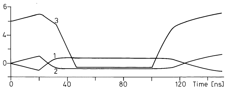
Fig 7.4: Cl.v = 1, Cemit.V = 2, Ccoll.V = 3
